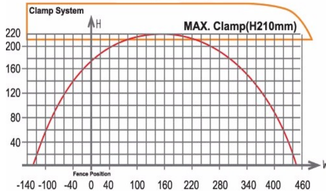
CS-24L Cutting Capacity Chart
